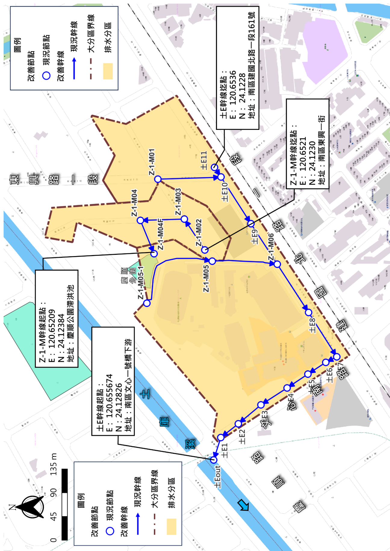
三、Z-1-M 幹線及土 E 幹線排水區域範圍圖
