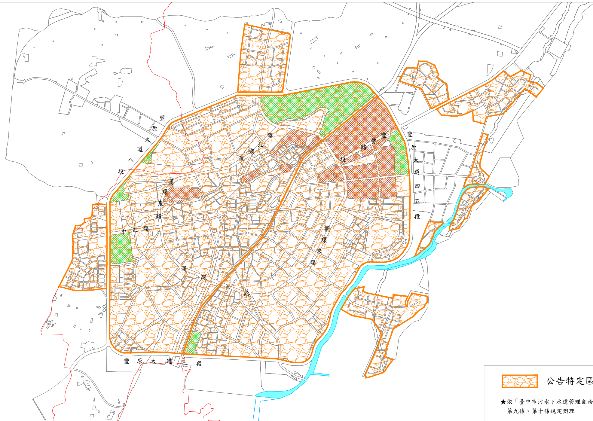
臺中市污水下水道用戶排水設備審查區域示意圖-豐原系統
