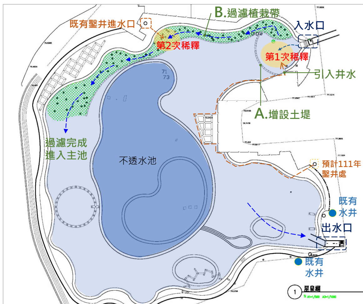
圖 19 星泉湖過濾系統初步規劃配置
