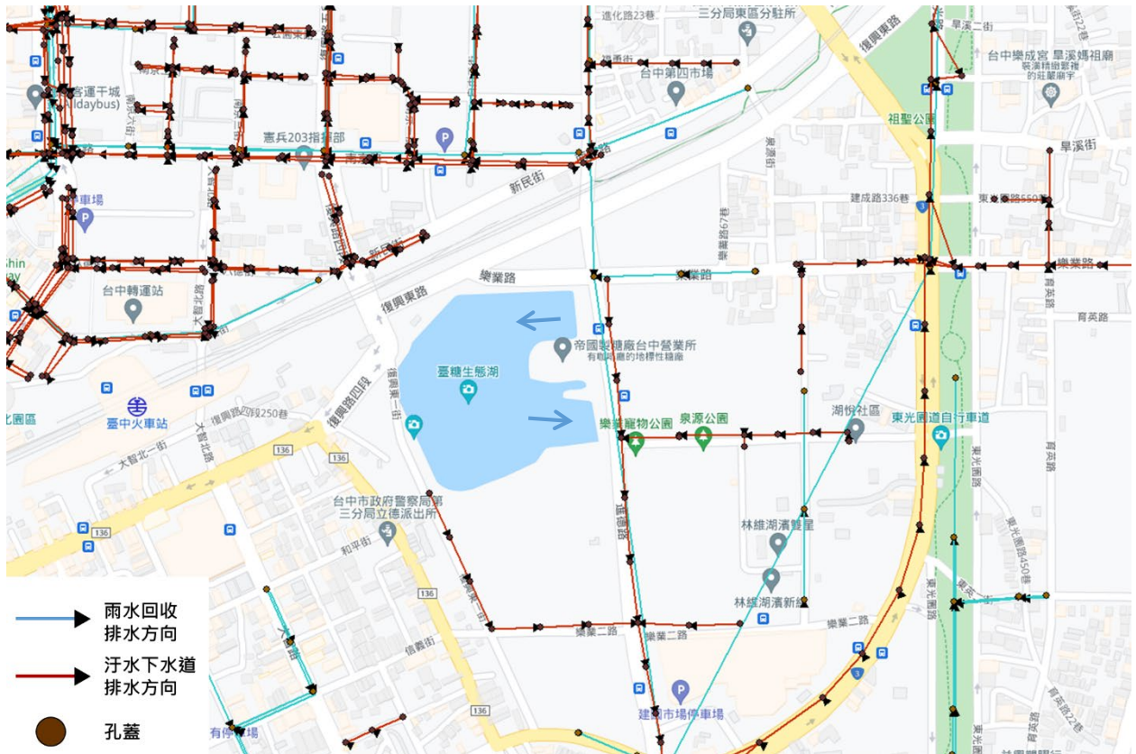
圖 11 星泉湖周邊地下管線分布圖
