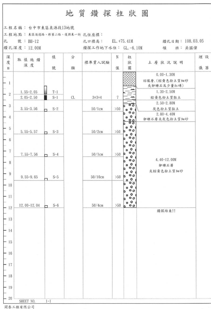
圖 15 地質鑽探柱狀圖
