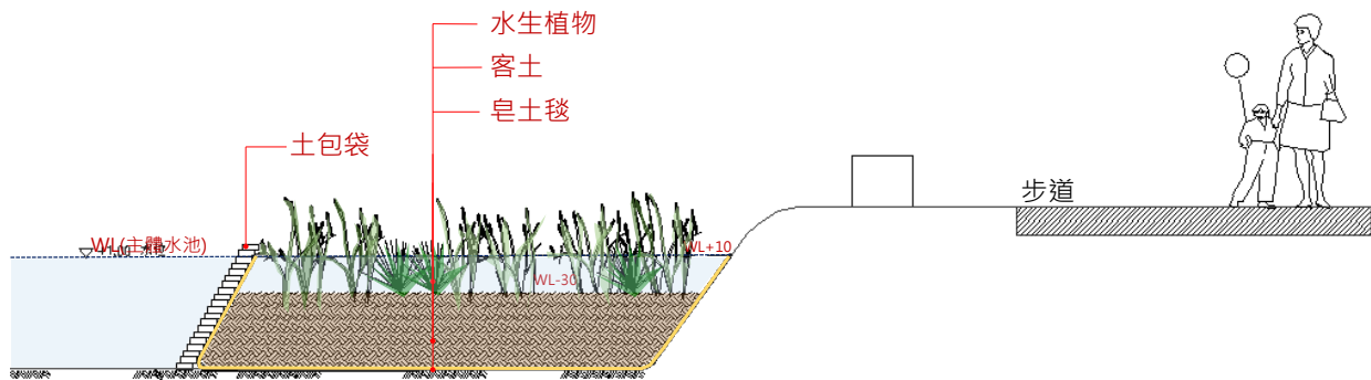
圖 20 過濾系統剖面示意圖
